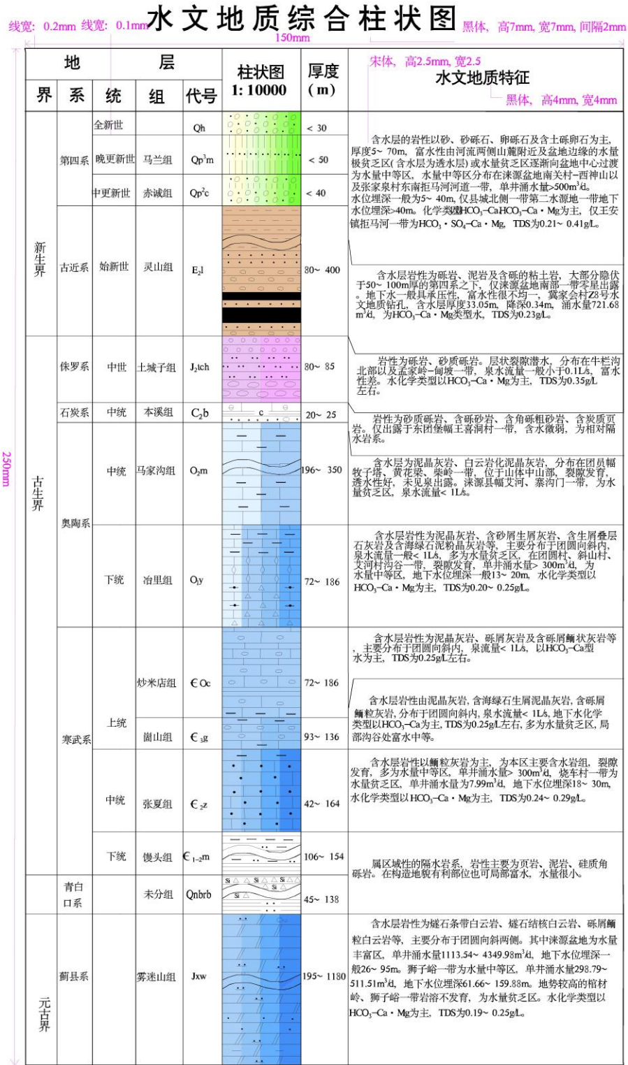
图A.3 水文地质综合柱状图
