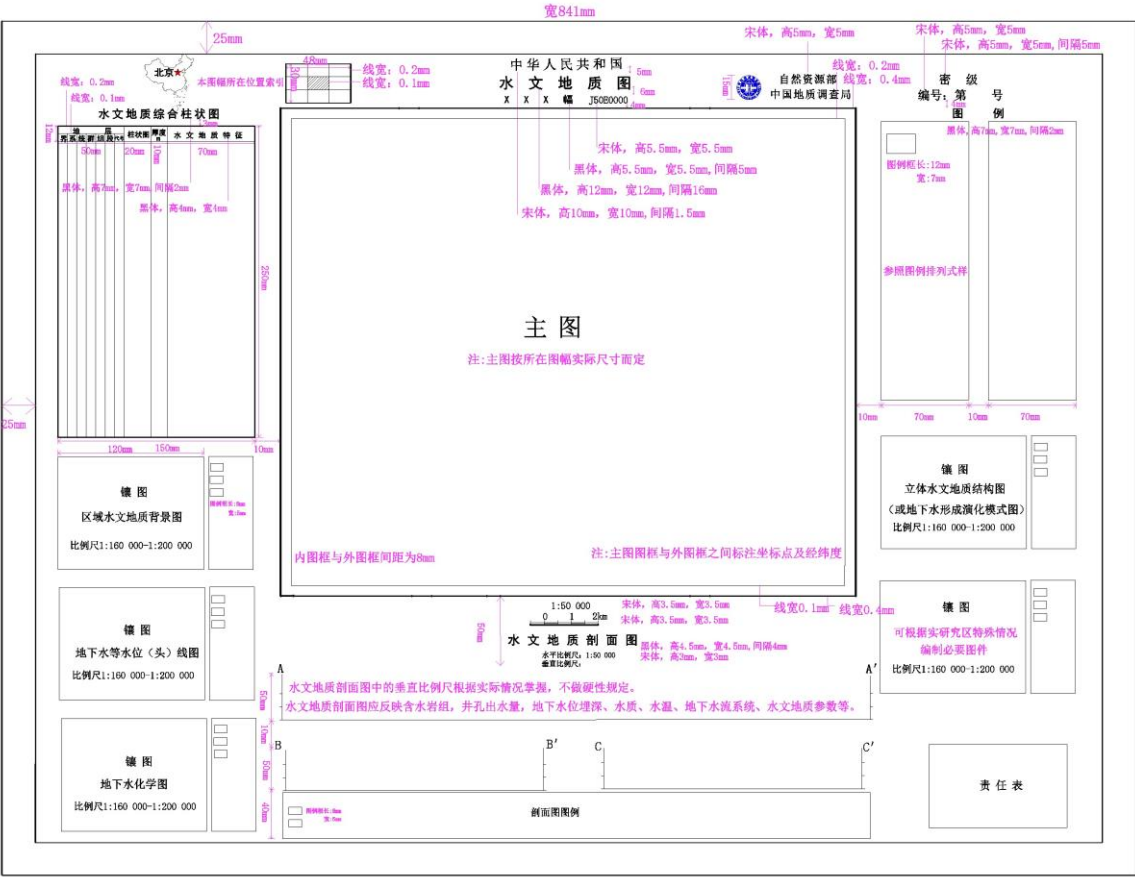
图A.1 标准图幅水文地质图图面配置
